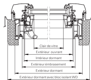
Coupe B-B
