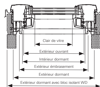
Coupe B-B
